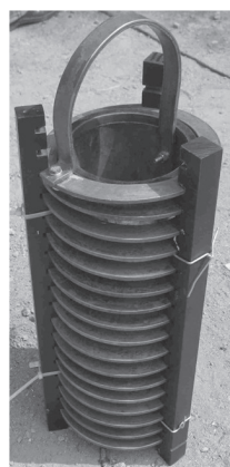
Componenta de luptă convențională pentru generarea unui puls electromagnetic destinat blocării sistemelor C4 I
